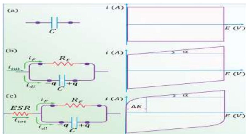
شکل (۱۰-۱) شماتیک مدار معادل و منحنی ولتاژ و ولتاژ چرخه‌ای مرتبط با آن [۲]
