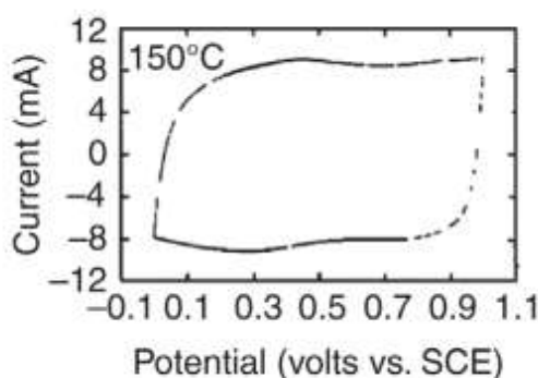
شکل ۲-۱۸-ولتاموگرام چرخه ای \text{RuO}_2 \cdot x\text{H}_2\text{O}
