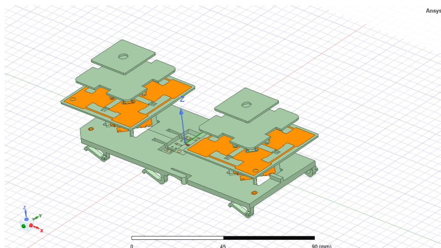
شکل ۷: مدل سازی نمونه آنتن ۵G
