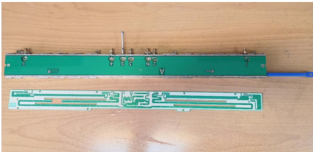
شکل ۵: ساخت یک نمونه از فیز شیفتر با استفاده فیبر مدار چاپی به جای آلومینیوم
