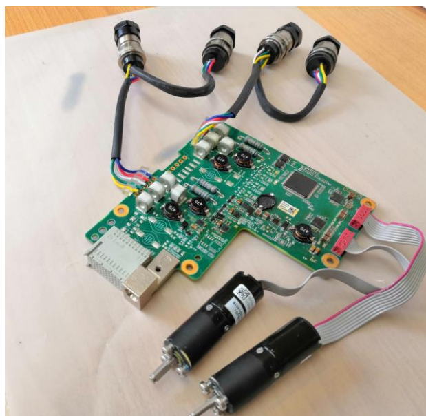
شکل ۱: نمونه برد الکترونیکی RET به همراه موتور ها
