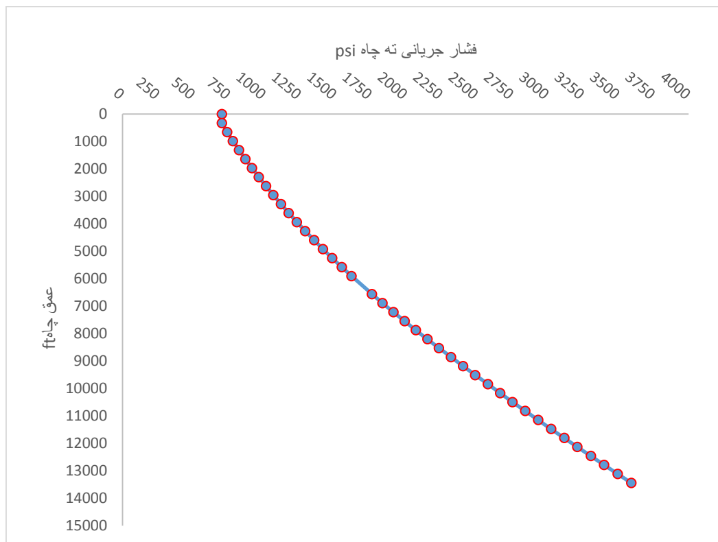
شکل شماره ۶: نمودار فشار جریان ته چاه در مقابل عمق
