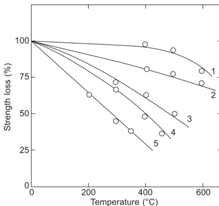
شکل ۱- اثر اجزای شیمیایی تشکیل دهنده شیشه بر استحکام الیاف شیشه پس از عملیات حرارتی: ۱. کوارتز؛ ۲. سیلیکا؛ ۳. آلومینوم بوروسیلیکات عاری از قلیا؛ ۴. سیلیکات کلسیم سدیم؛ ۵. بورات [۲].
